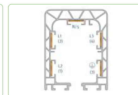
Вид в разрезе/расположение шин
